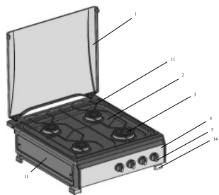
Рисунок 3 Плита газовая бытовая четырёхгорелочная ПГ4 1469 (настольный вариант, тип ANG)
